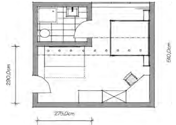
Grundriss eines hochwertig umgebauten Pensionszimmer mit optimaler Ausnutzung der vorhandenen räumlichen Gegebenheiten.
